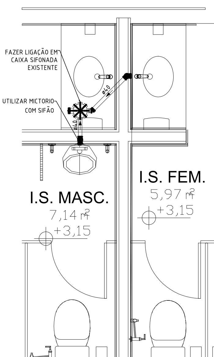
DETALHE 05 ESCALA 1:25
