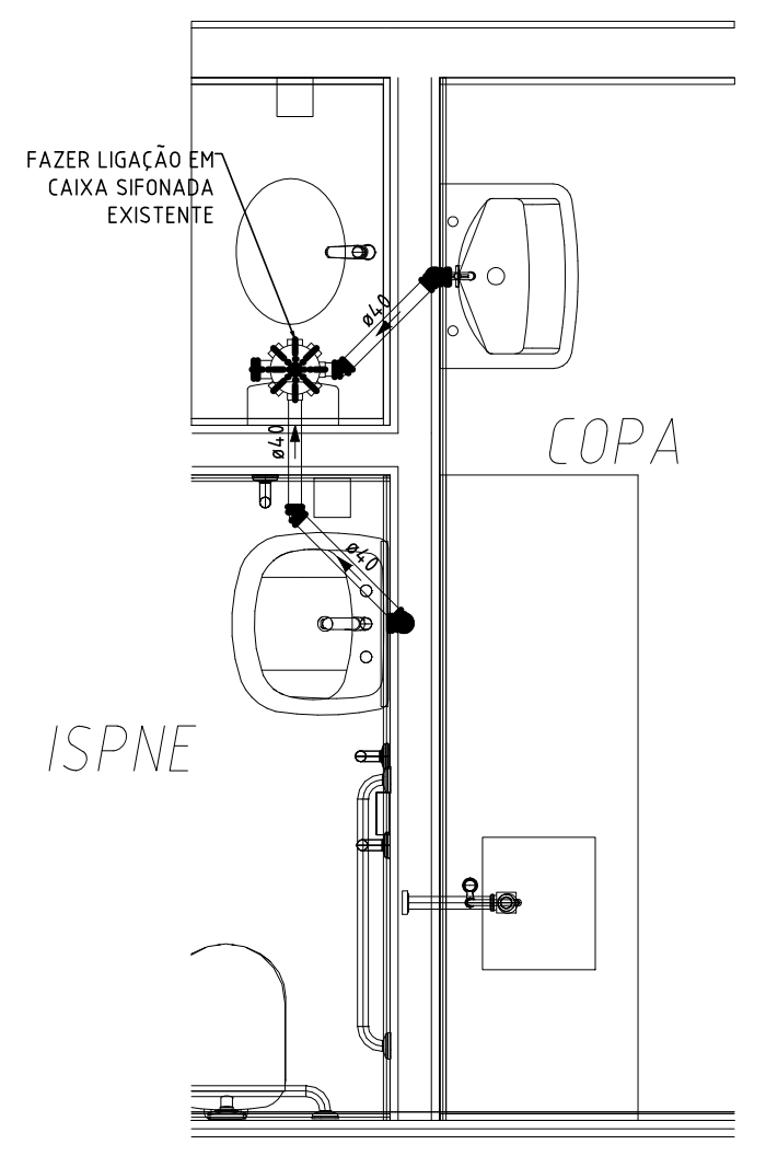
DETALHE 04 ESCALA 1:25
